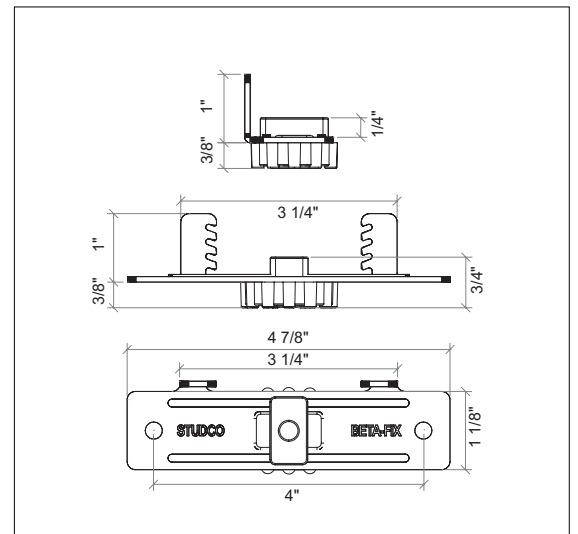
MBFR DIMENSIONS
